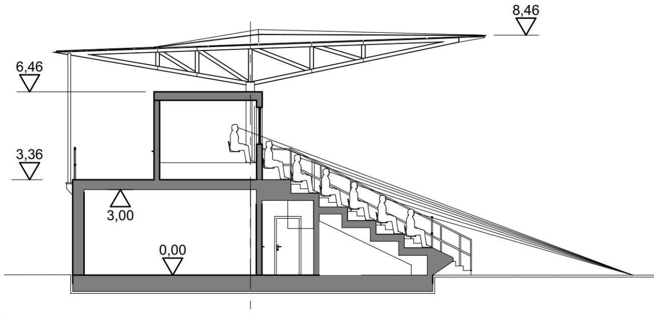
PRZEKRÓJ POPRZECZNY
